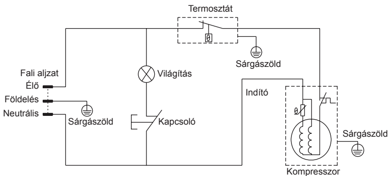
Bekapcsolási ábra
